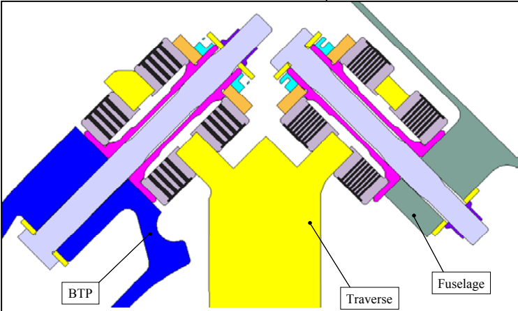
Section de la liaison BTP – Traverse - Fuselage
