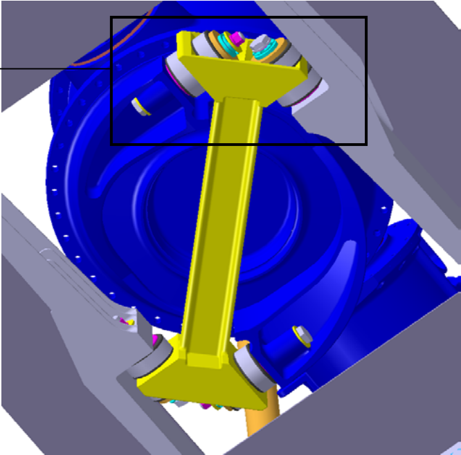
Section de la liaison BTP – Traverse - Fuselage
